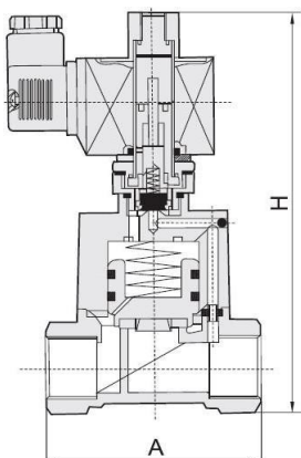
Рисунок 1. Эскиз
